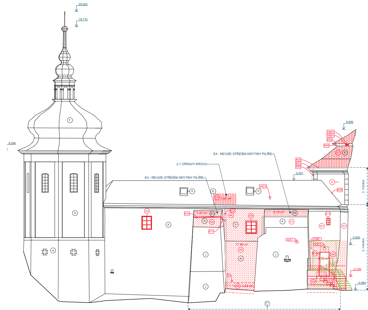
5 - JIŽNÍ POHLED
