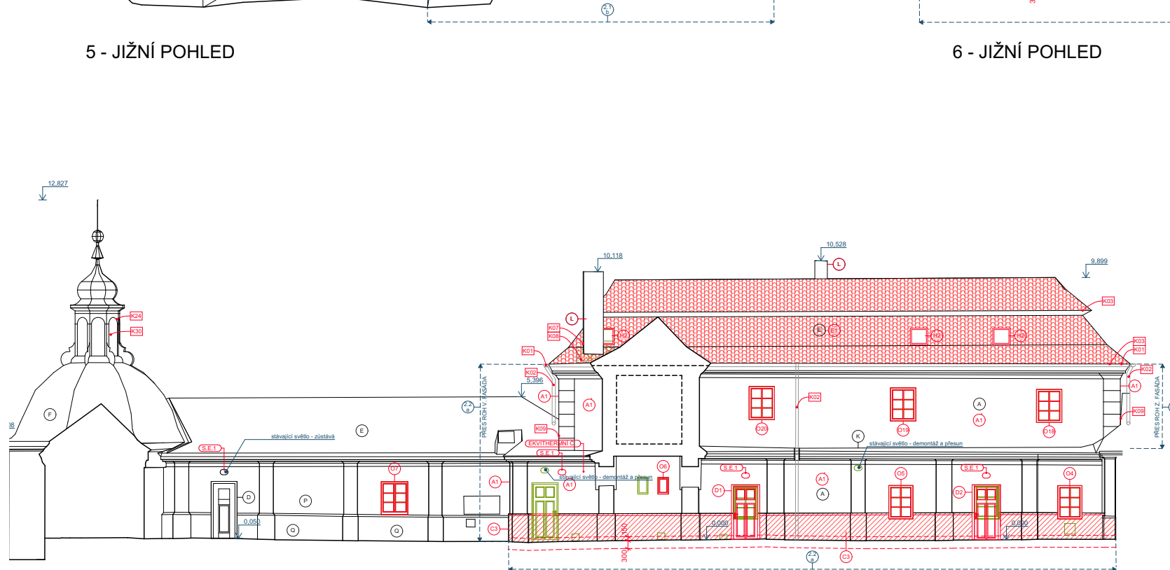
7 - SEVERNÍ POHLED
