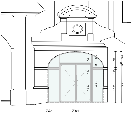
POHLED VÝCHODNÍ M 1:50
