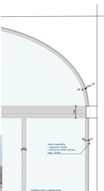
DETAIL OSTĚNÍ M 1:10
