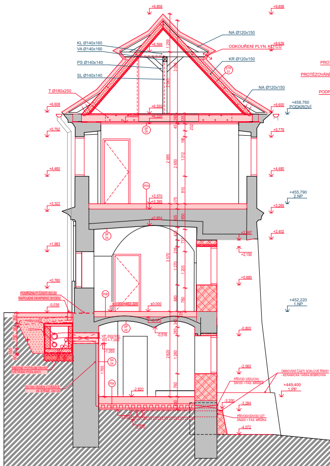
ŘEZ B - SO.2
