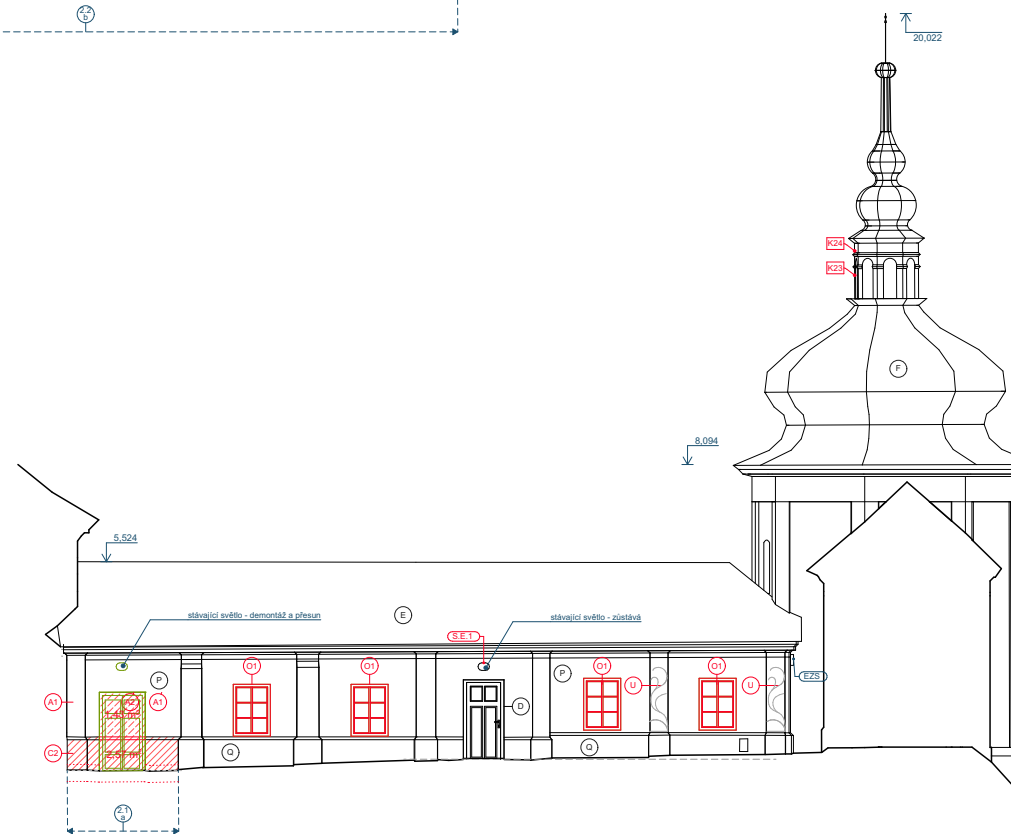
8 - SEVERNÍ POHLED
