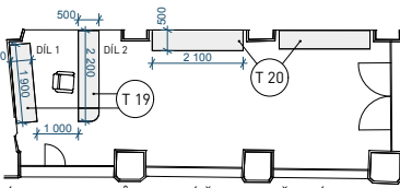
INFOCENTRUM - CELKOVÝ PŮDORYS M 1:100
