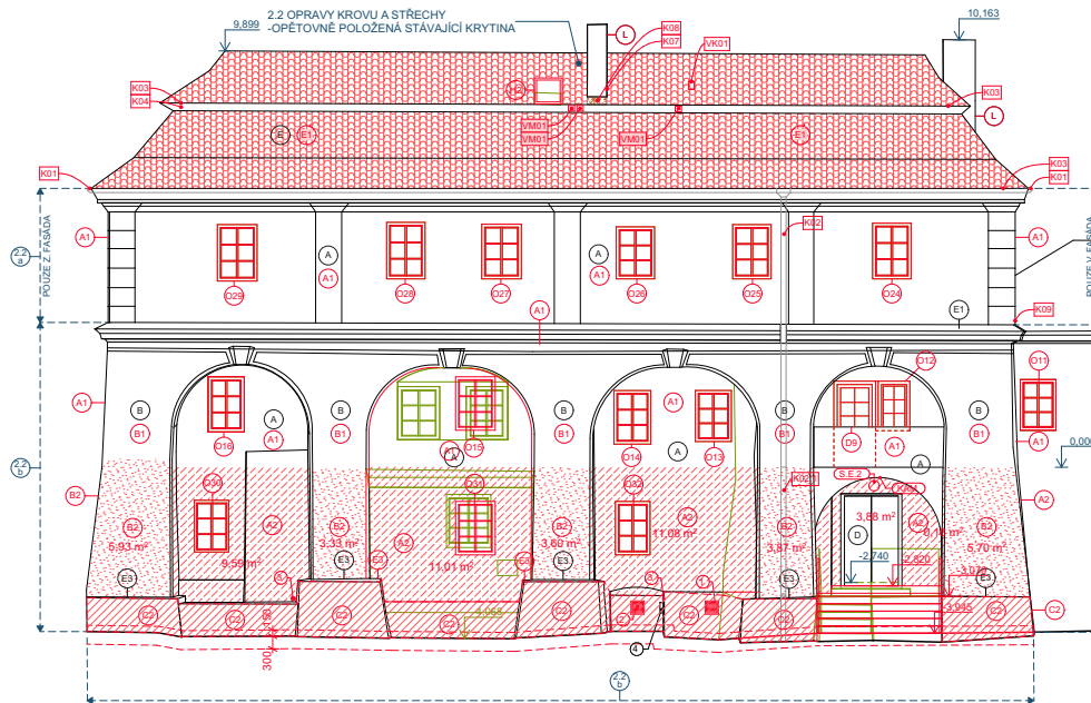
6 - JIŽNÍ POHLED
