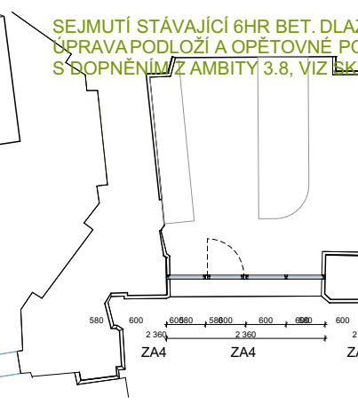
PŮDORYS INFOCENTRA M 1:50
