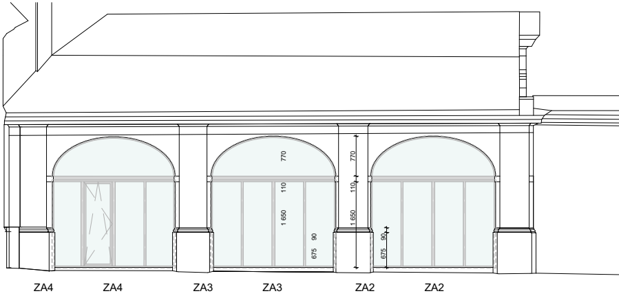
POHLED JIŽNÍ AMBITY INFOCENTRA M 1:50
