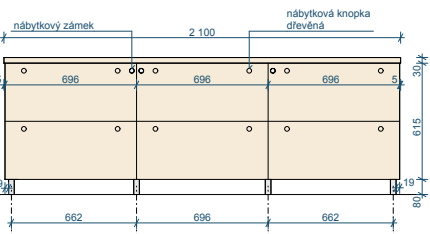
T 20 POHLED ČELNÍ M 1:20
