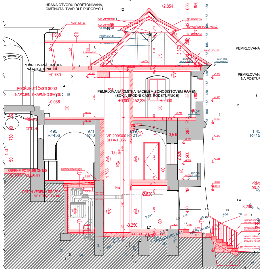
ŘEZ C - SO.2
